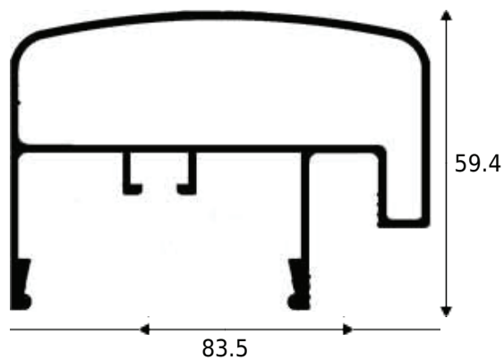
CG-083 1,334 KG/M
