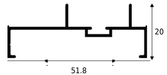
MB-004 0.276 KG/M
