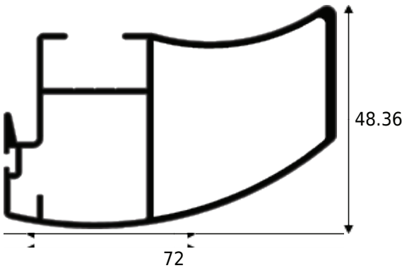
SI-2539 0.992 KG/M
