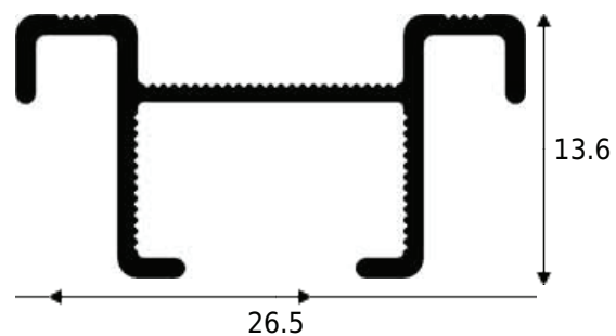
PF2-BL16 0.160 KG/M
