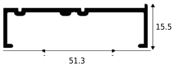
MB-003 0.287 KG/M
