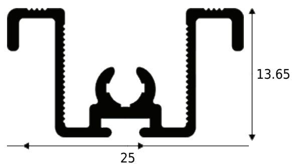
JHPF6-BL16 0.199 KG/M
