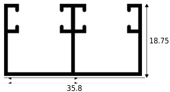
KP-063 0.298 KG/M
