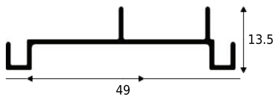
PF2-JL14 0.249 KG/M
