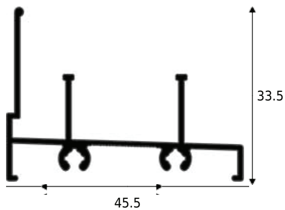
KDK-006 0.355 KG/M
