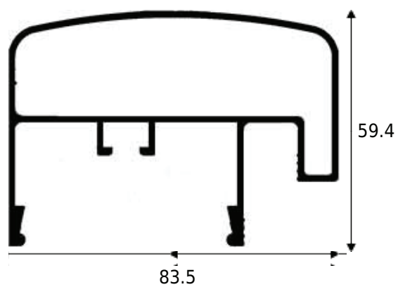
CG-083 1,334 KG/M
