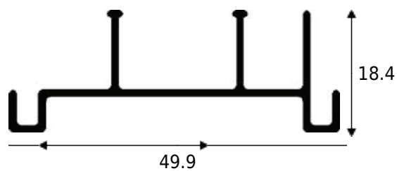
PF4-JL14 0.284 KG/M
