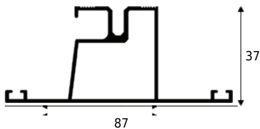
MAN-009 0.855 KG/M
