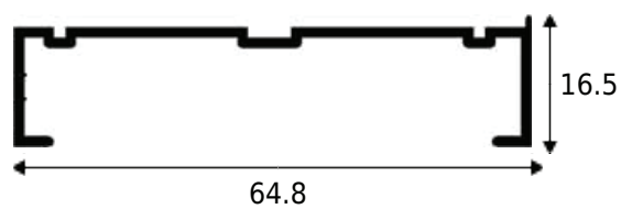
MP-397 0.379 KG/M
