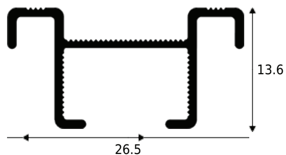
JHPF2-BL16 0.147 KG/M
