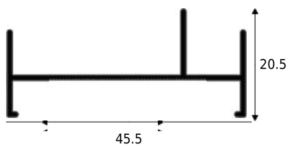
KDK-004 0.209 KG/M
