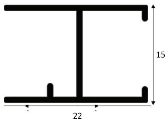
KDK-002 0.152 KG/M
