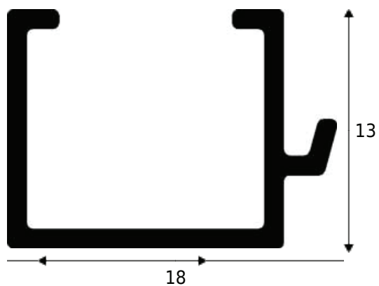
PF5-JL14 0.127 KG/M
