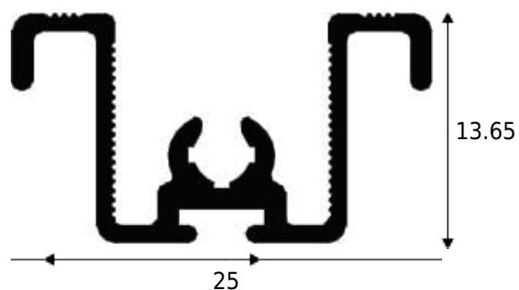
PF6-BL16
